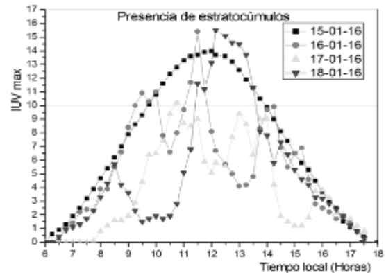
Figura 14. Presencia de nubes estratocúmulos se nota que los valores del IUV máximo diario a un día sin nubes
