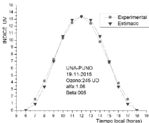
Figura 5. Índice UV experimental y estimado para 19 de noviembre 2015
