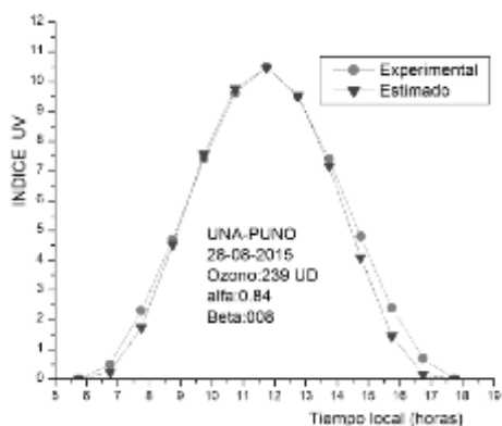
Figura 3. IUUV experimental y estimado para 28 de agosto 2015 El valor del IUUV máximo diario calculado para el día 9 de octubre del 2015 se presenta a las 12 pm y es de 13, valor que correspondería a un nivel de riesgo extremadamente alto según la escala de la OMS (Figura 4).
