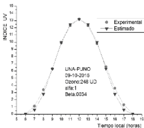
Figura 4. Índice UV experimental y estimado para 9 de octubre 2015
