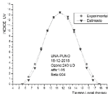
Figura 6. Índice UV experimental y estimado para 15 de diciembre 2015
