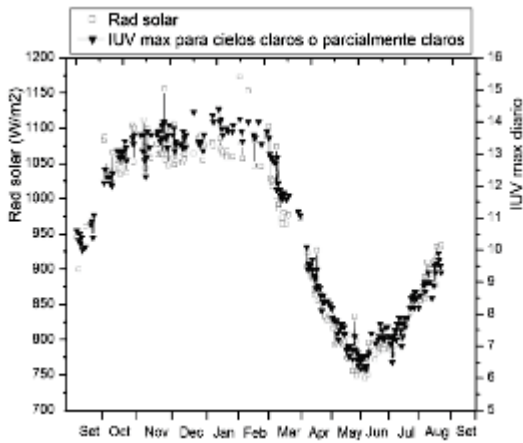
Figura 11. Comparación diaria de la radiación solar y el IUV máximo diario. Para cielos sin nubes o nublados antes o después del mediodía
