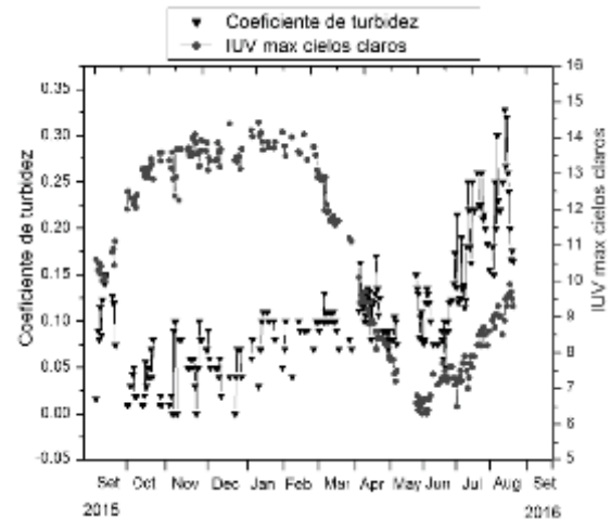
Figura 13. Influencia atmosférica del coeficiente de turbidez sobre el IUV máximo diario
