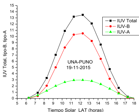
Figura 8. Porcentaje para el IUV máximo al medio día solar
