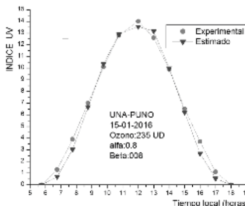
Figura 7. Índice UV experimental y estimado para 15 de enero 2016
