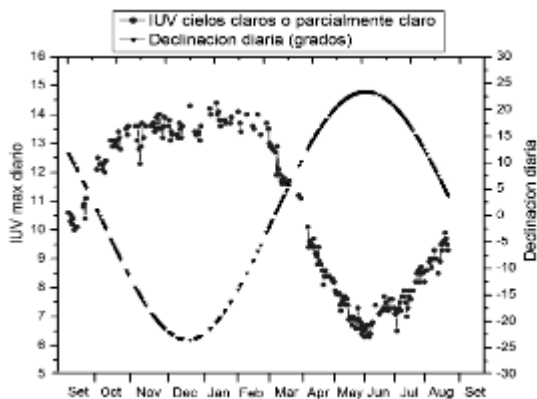
Figura 12. Influencia del factor geométrico declinación del sol sobre el IUV máximo diario en la superficie terrestre
