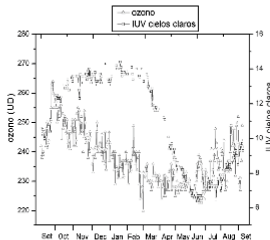
Figura 10. Influencia atmosférica del Ozono sobre el IUV máximo diario
