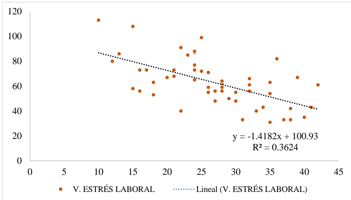
Figura de regresión lineal MCO
