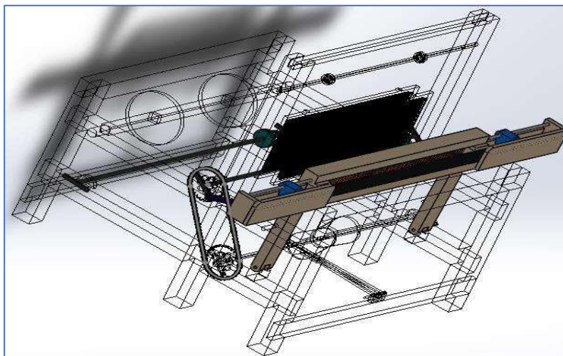
Figura 11: Sistema del batán del prototipo.
