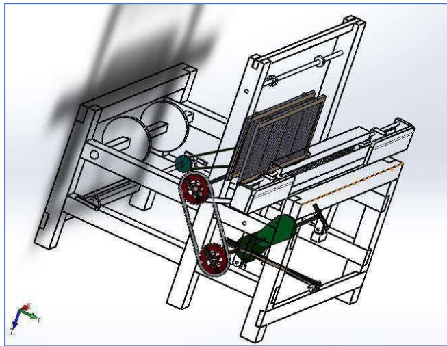
Figura 9: Sistema de pedales del telar prototipo.
