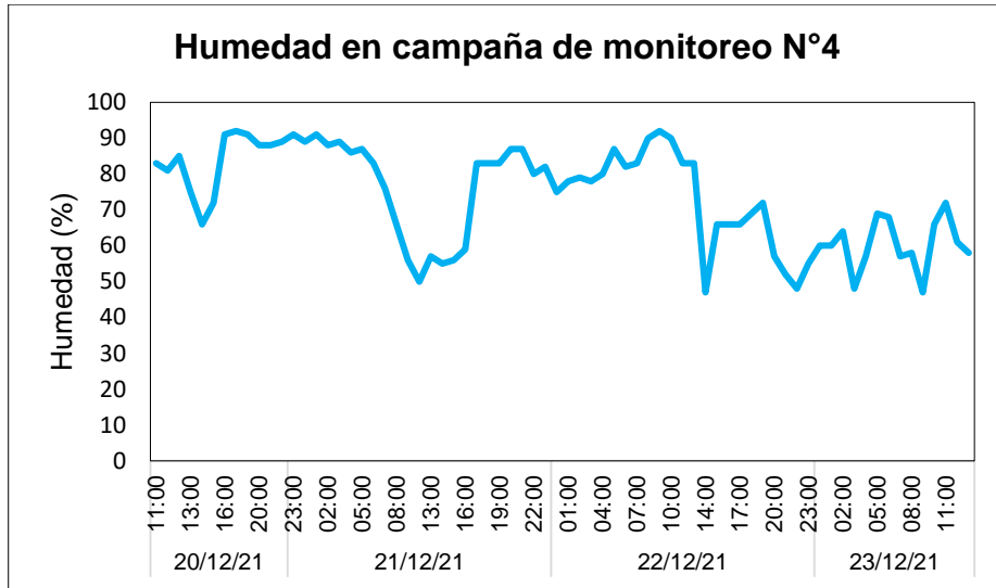
Figura 45. Comportamiento de la humedad en campaña de monitoreo N°4
