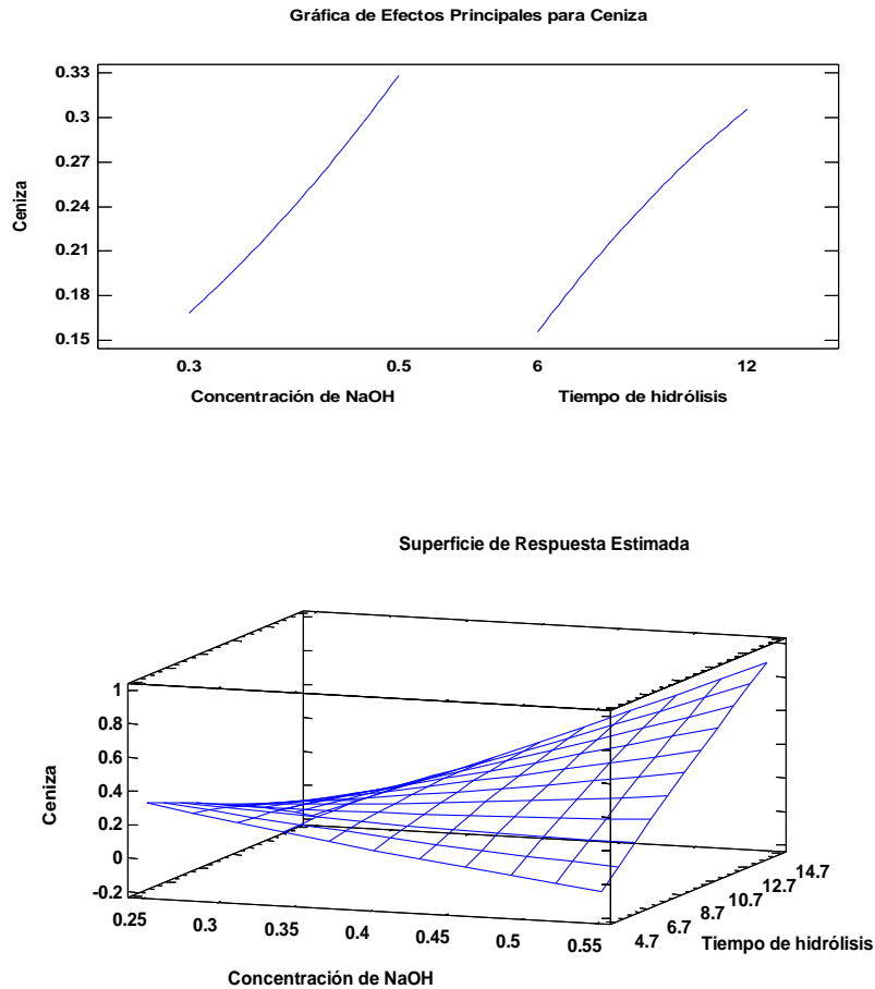
Figura 13: Gráfico de efectos principales y superficie de respuesta de la ceniza
