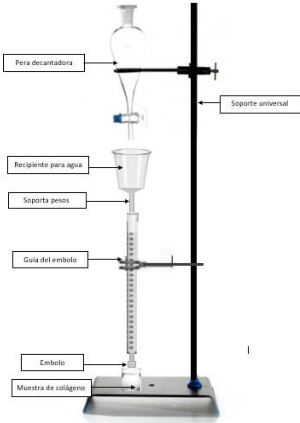
Figura 7: Diseño del dispositivo para medir la fuerza gel del colágeno
