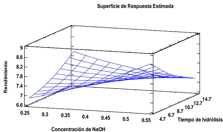
Figura 9: Superficie de respuesta estimada del rendimiento
