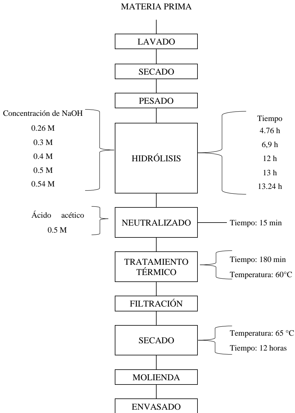
Figura 5: Diagrama de flujo para la extracción del colágeno
