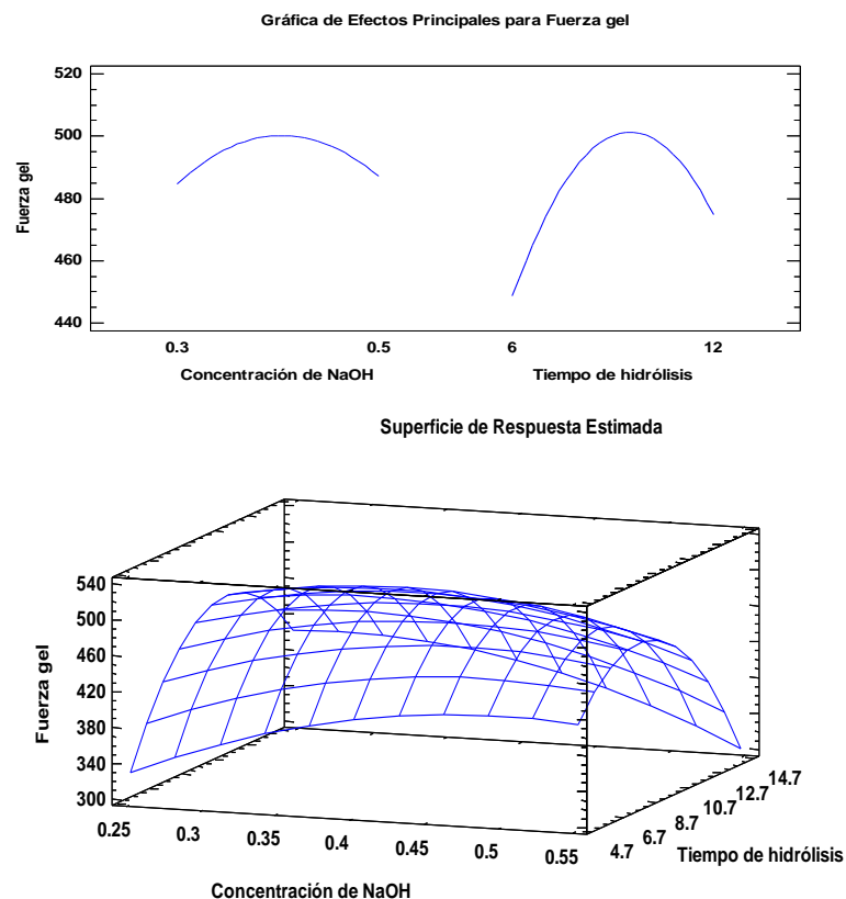
Figura 10: Efectos principales y superficie de respuesta estimada de fuerza gel.
