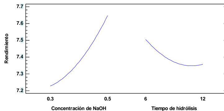
Figura 8: Efectos principales del rendimiento
