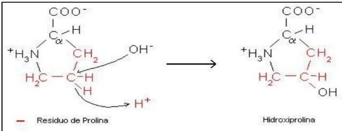
Figura 3: Fórmula estructural de la prolina e hidroxiprolina
