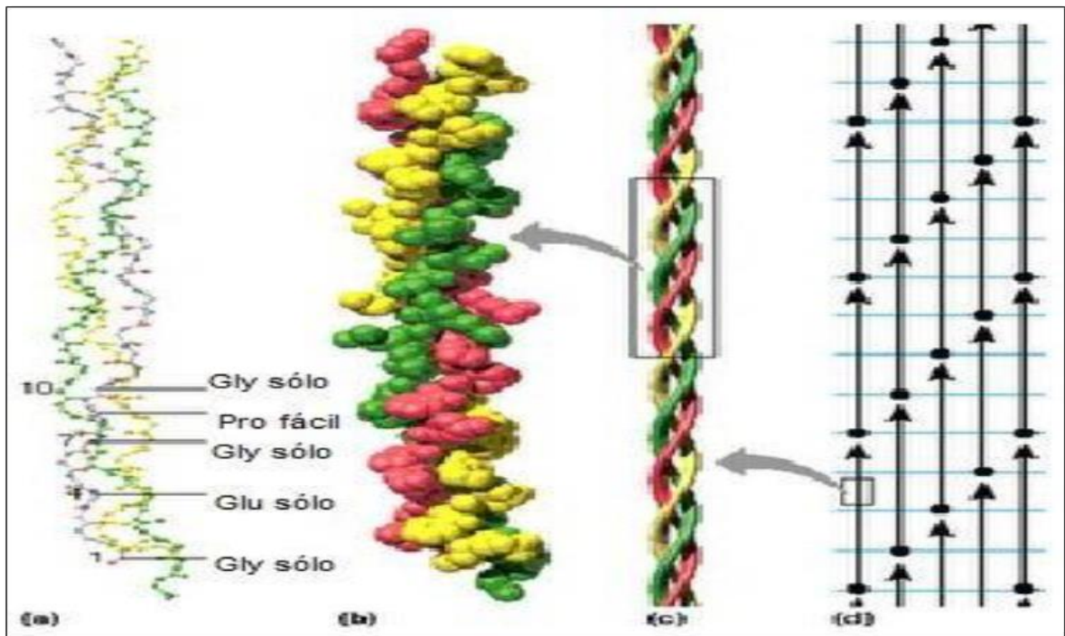
Figura 4: Representación esquemática de la molécula del colágeno
