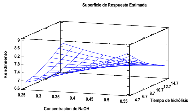
Figura 9: Superficie de respuesta del rendimiento
