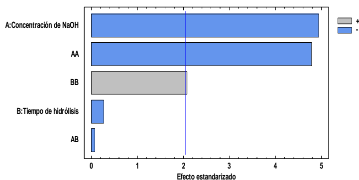
Diagrama de Pareto Estandarizada para Humedad
