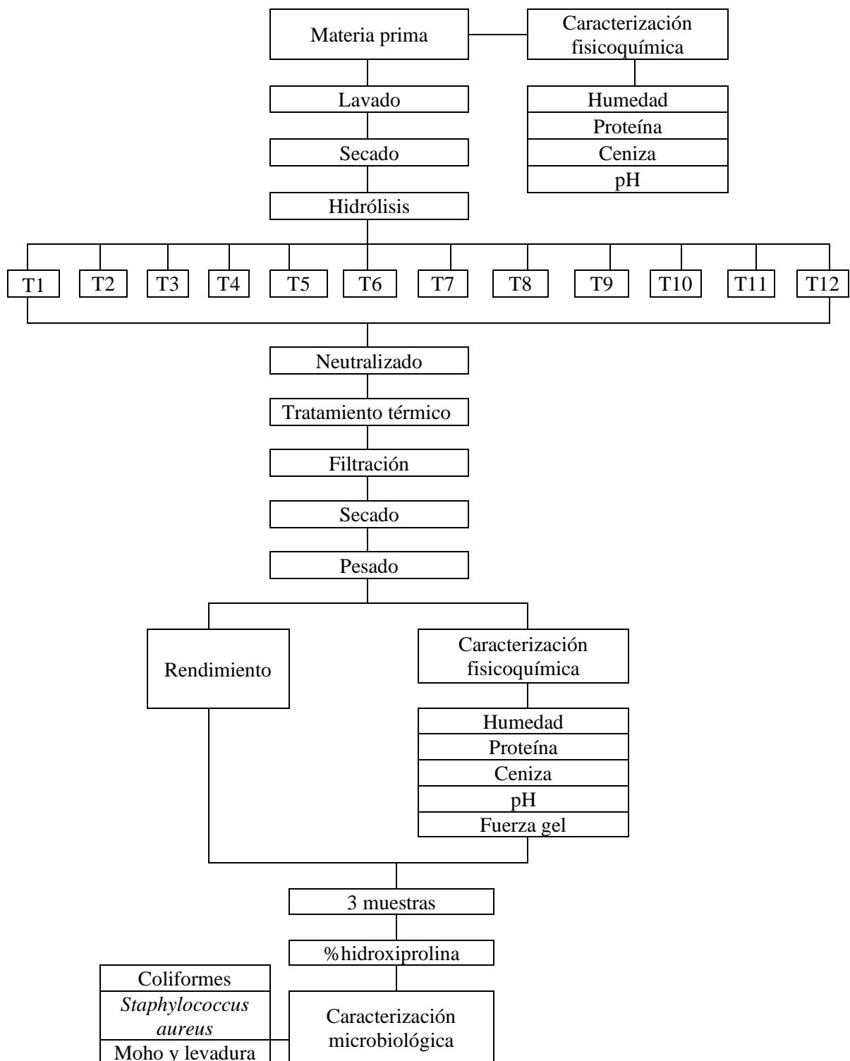
Figura 6: Diseño experimental de la extracción de colágeno
