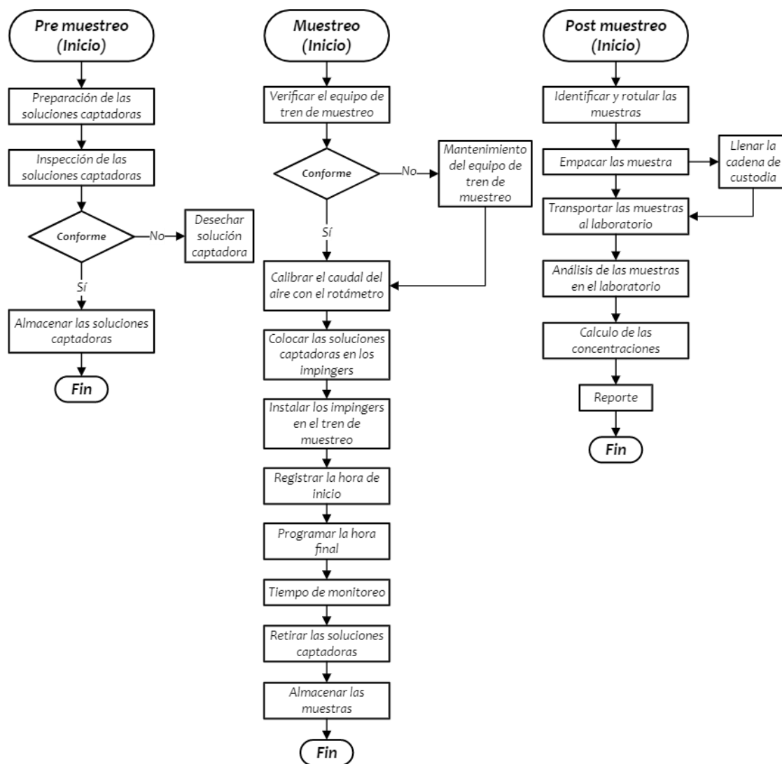
Figura 5. Etapas del muestreo de SO 2 , NO 2 , CO y O 3
